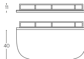
pianta/plan
