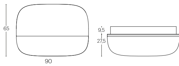
fronte/front
